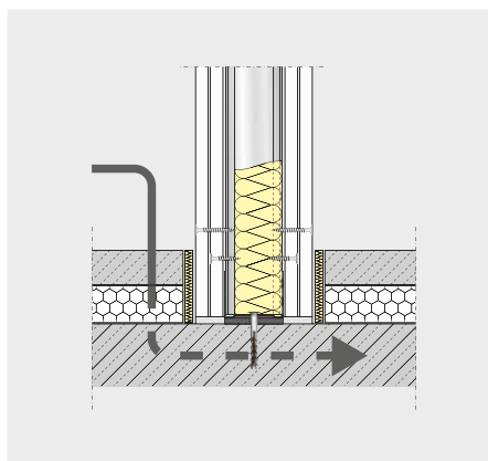
Fußbodenaufbau unterbrochen
