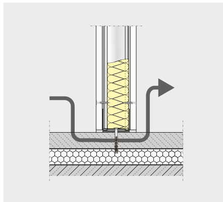
Durchgehender Fußbodenaufbau
